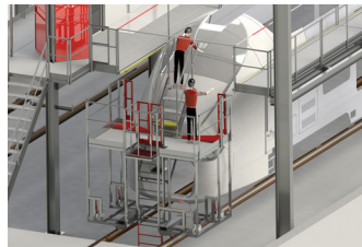
Plateforme d'accès au pare-brise.
